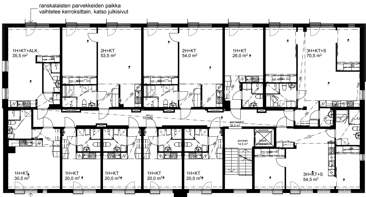
B-PORRAS 2.-5. KERROS
